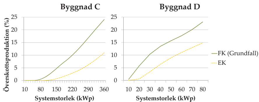
Figur 10 Överskottsproduktion för byggnad C och D för två olika fall: grundfallet med fjärrkyla (FK) samt det alternativa fallet med eldriven kylmaskin (EK).
