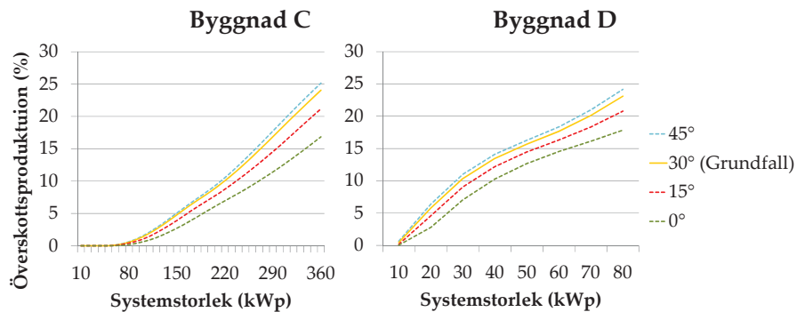
Figur 16 Överskottsproduktion för byggnad C och D för söderriktade solceller i 45°, 30°, 15° och 0° lutning.
