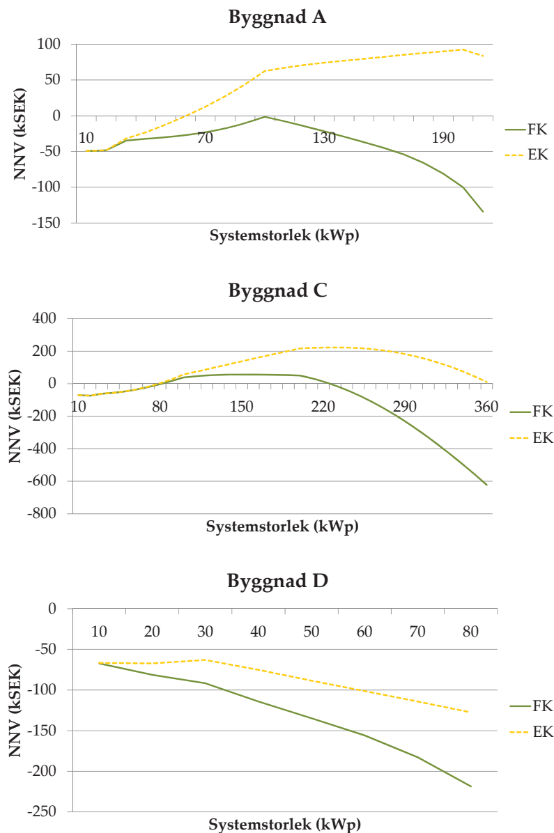
Figur 20 Nettonvärdet för byggnad A, C och D i grundfallet med fjärrkyla (FK) och i det alternativa fallet med eldriven kyla (EK) samt med ekonomiska förutsättningar givet referensscenariot.
