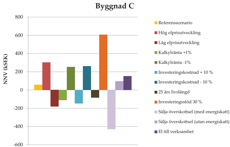
Figur 23 Nettonuvärde för solceller på byggnad C enligt grundfallet samt givet referensscenarioet och de alternativa ekonomiska scenarierna.
