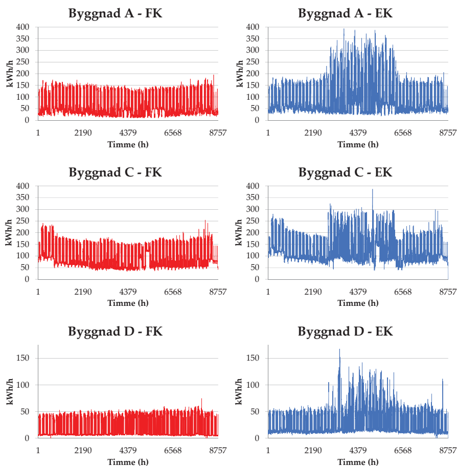
Figur 5 Elastprofil (fastighetsel) för byggnad A, C och D med antingen fjärrkyla (FK = röd) eller eldriven kyla (EK = blå) som kylsystem. Observera skillnaden i skala på y-axeln.
