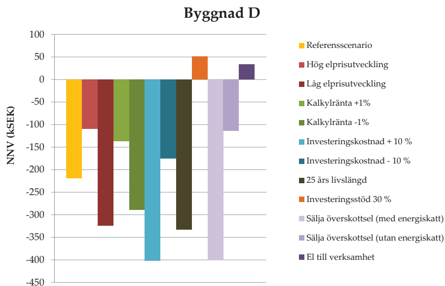
Figur 24 Nettonuvärde för solceller på byggnad D enligt grundfallet samt givet referensscenarioet och de alternativa ekonomiska scenarierna.
