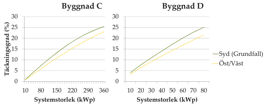
Figur 13 Täckningsgrad för byggnad C och D med takinstallerade solceller i 30° lutning riktade mot söder och öst/väst.
